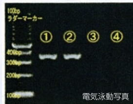
ノロウイルス陰性の場合には344dpの位置にバンドが出現
